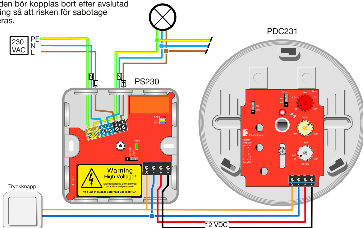
Principalschema för system PDC230.
